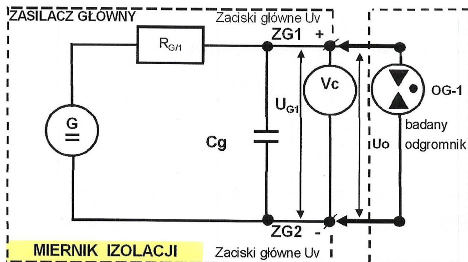
Rys. 10. Pomiar statycznego napięcia zapłonu odgromnika gazowego za pomocą układu generatora - zasilacza wolno narastającego napięcia, o regulowanym napięciu wyjściowym w zakresie (0 \div 500)\text{ V} i (0 \div 1000)\text{ V}
