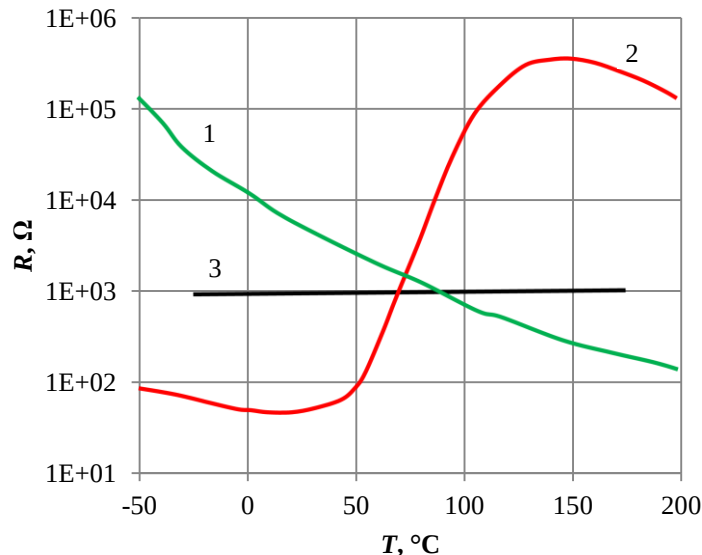
Rys. 2. Charakterystyka R = f(T) termistora typu NTC (1) oraz PTC (2) w odniesieniu do rezystora R (3)
